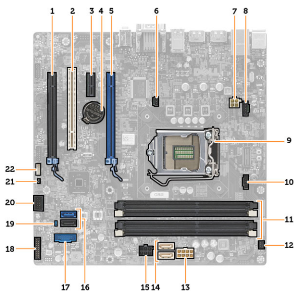
Skica 1. Komponente matične plošče
